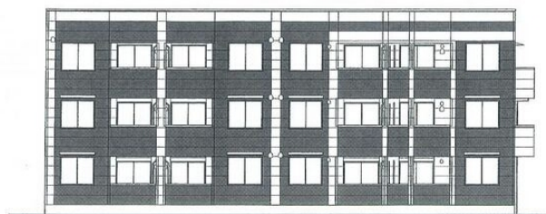
南 立面図 8=1:100
